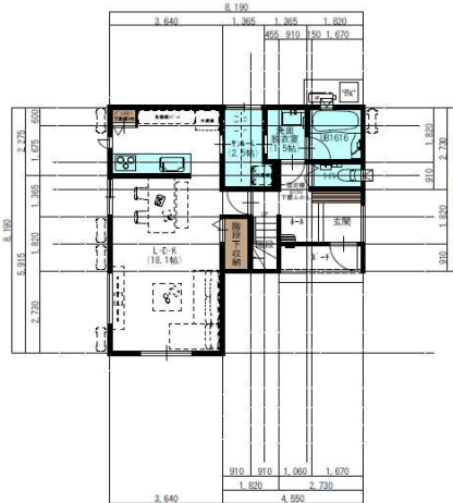
■ 1 階平面図 ■
